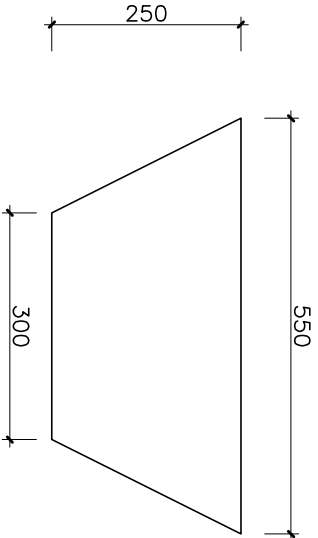
CORTE AA
